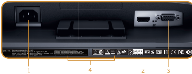
Veduta inferiore senza base del monitor
